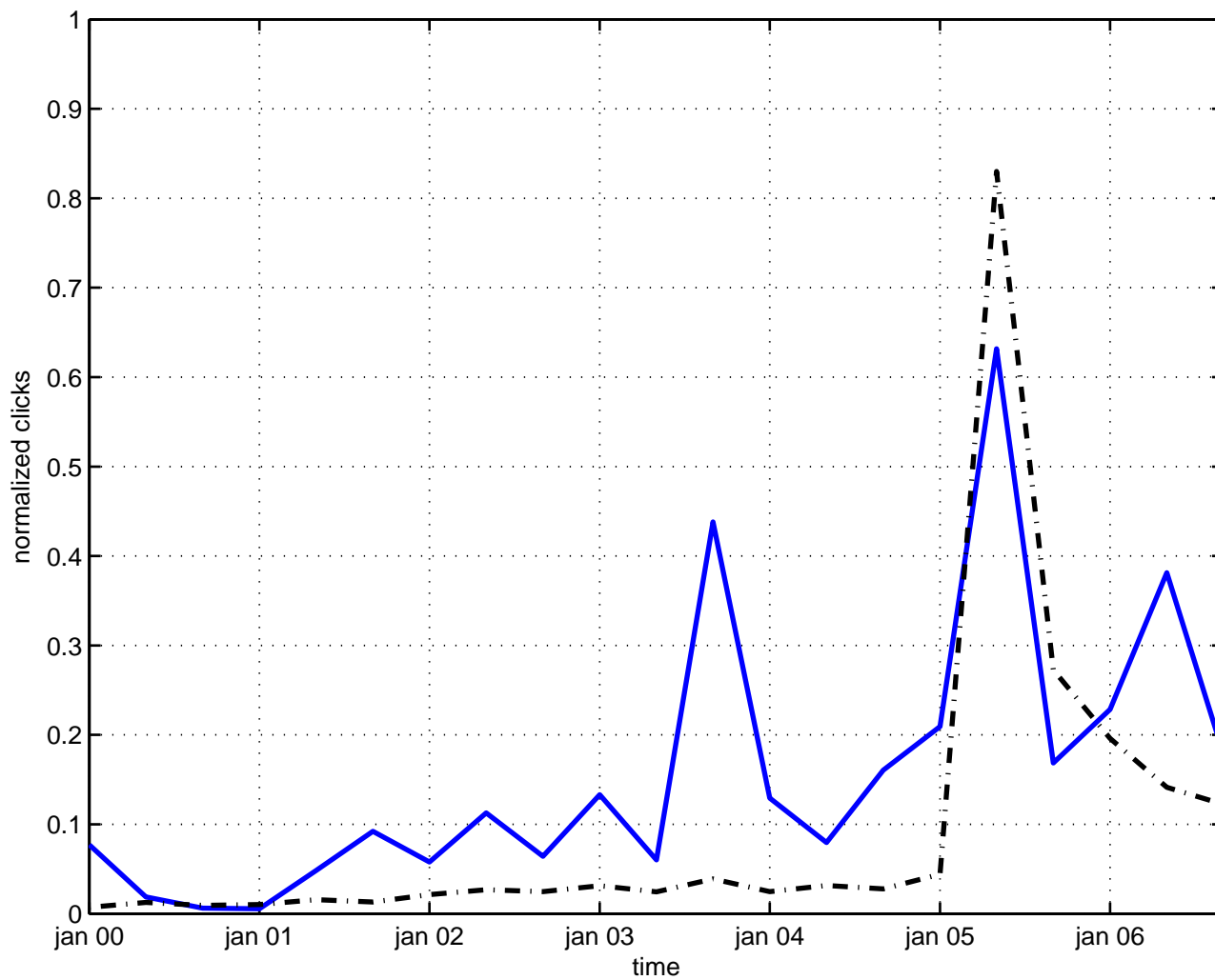
boson
