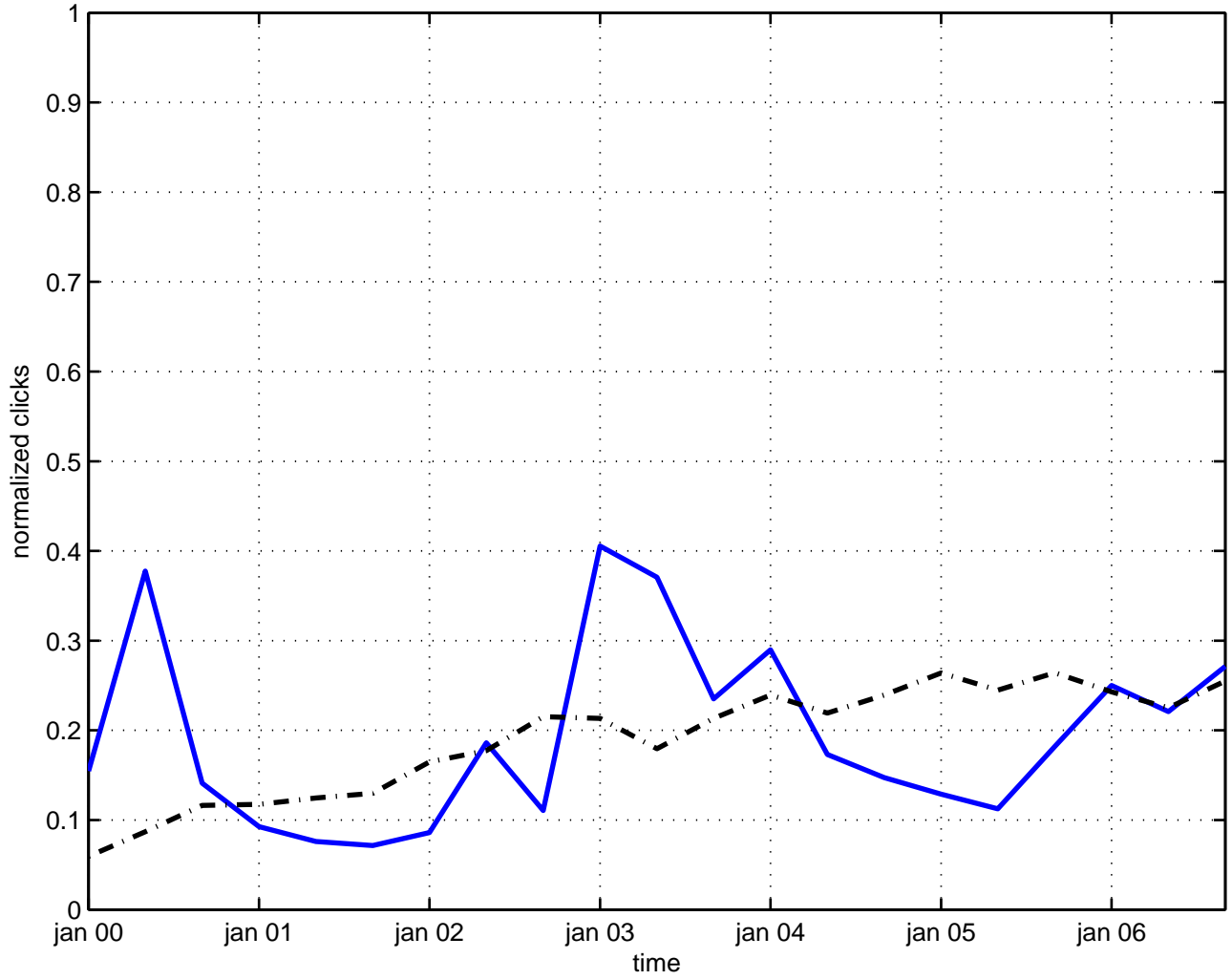
boson string
