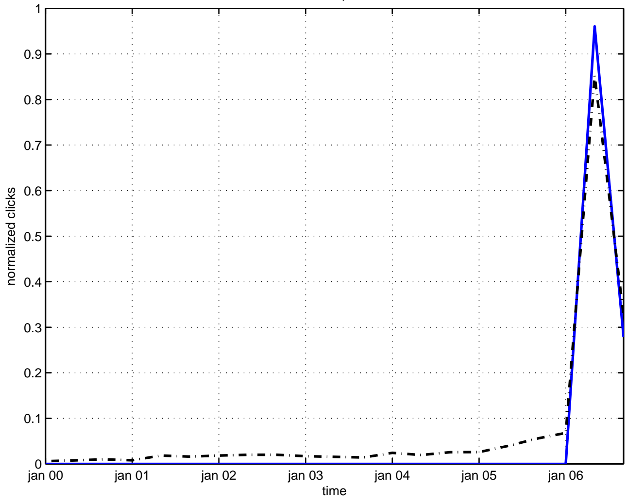
boson quark
