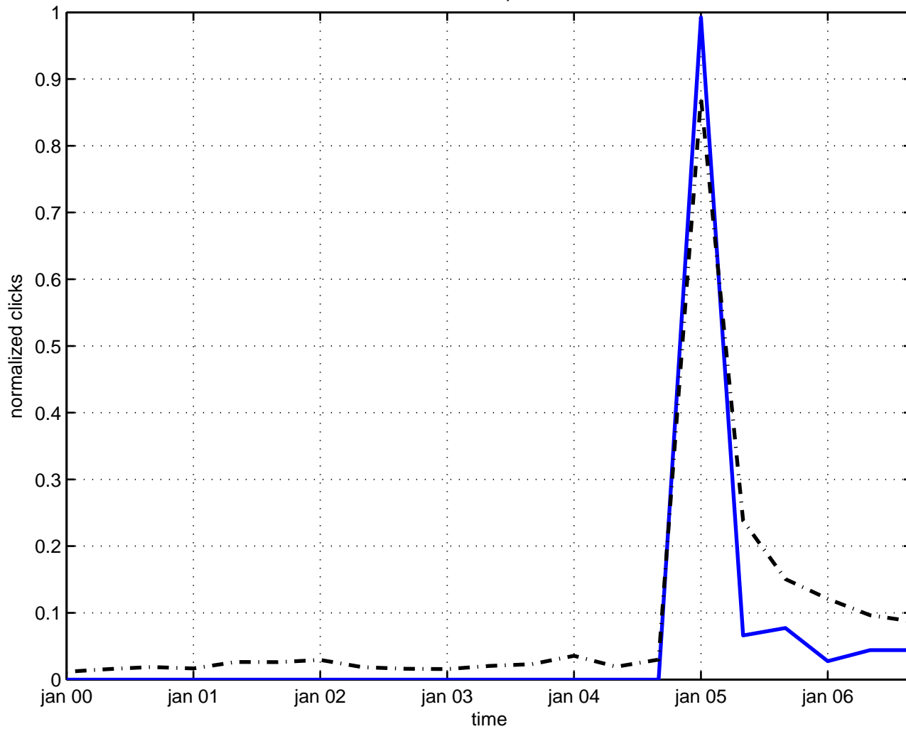
annihilation positron
