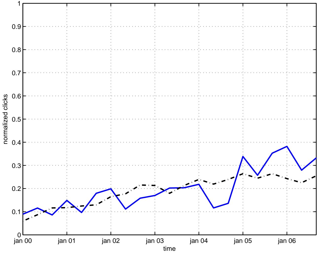
4 phi**n model
