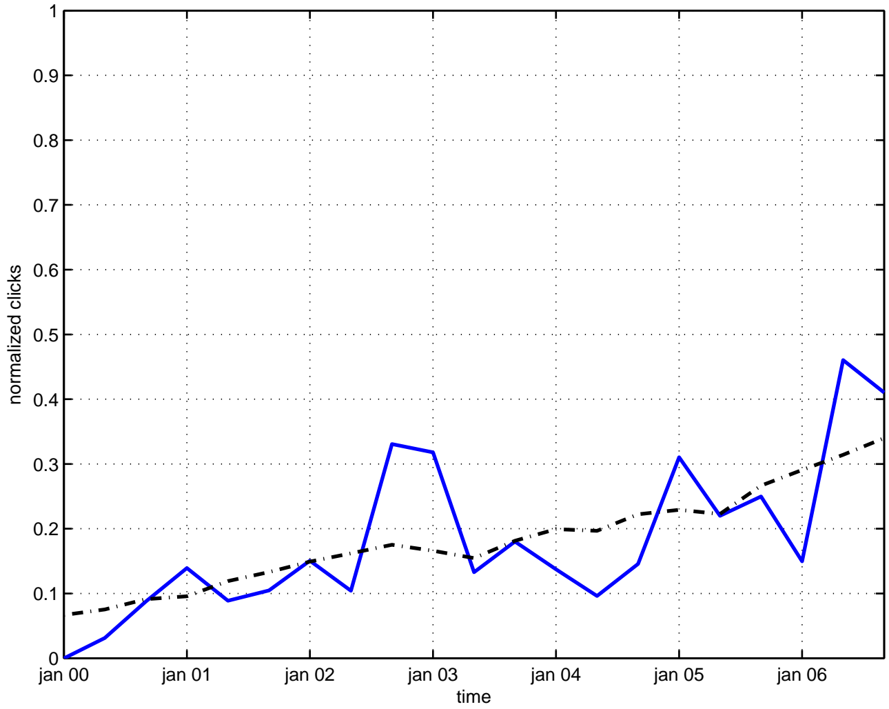
2 spin
