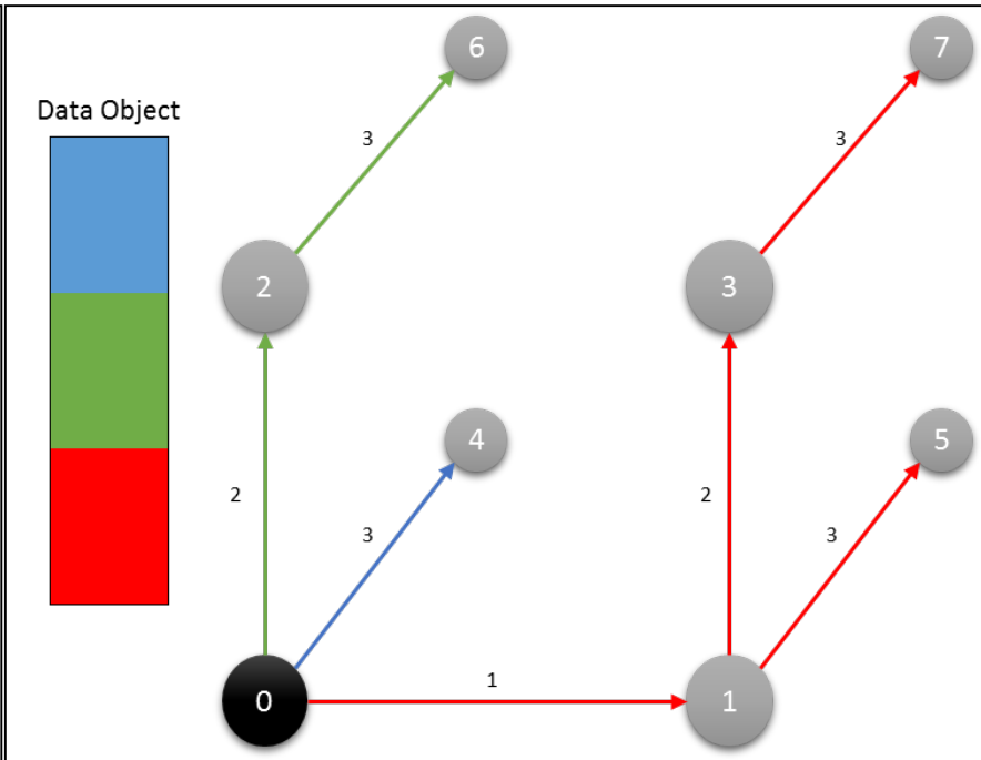
Binomial Pipeline
